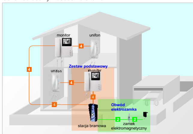
Schemat ideowy videodomofonu B/W
